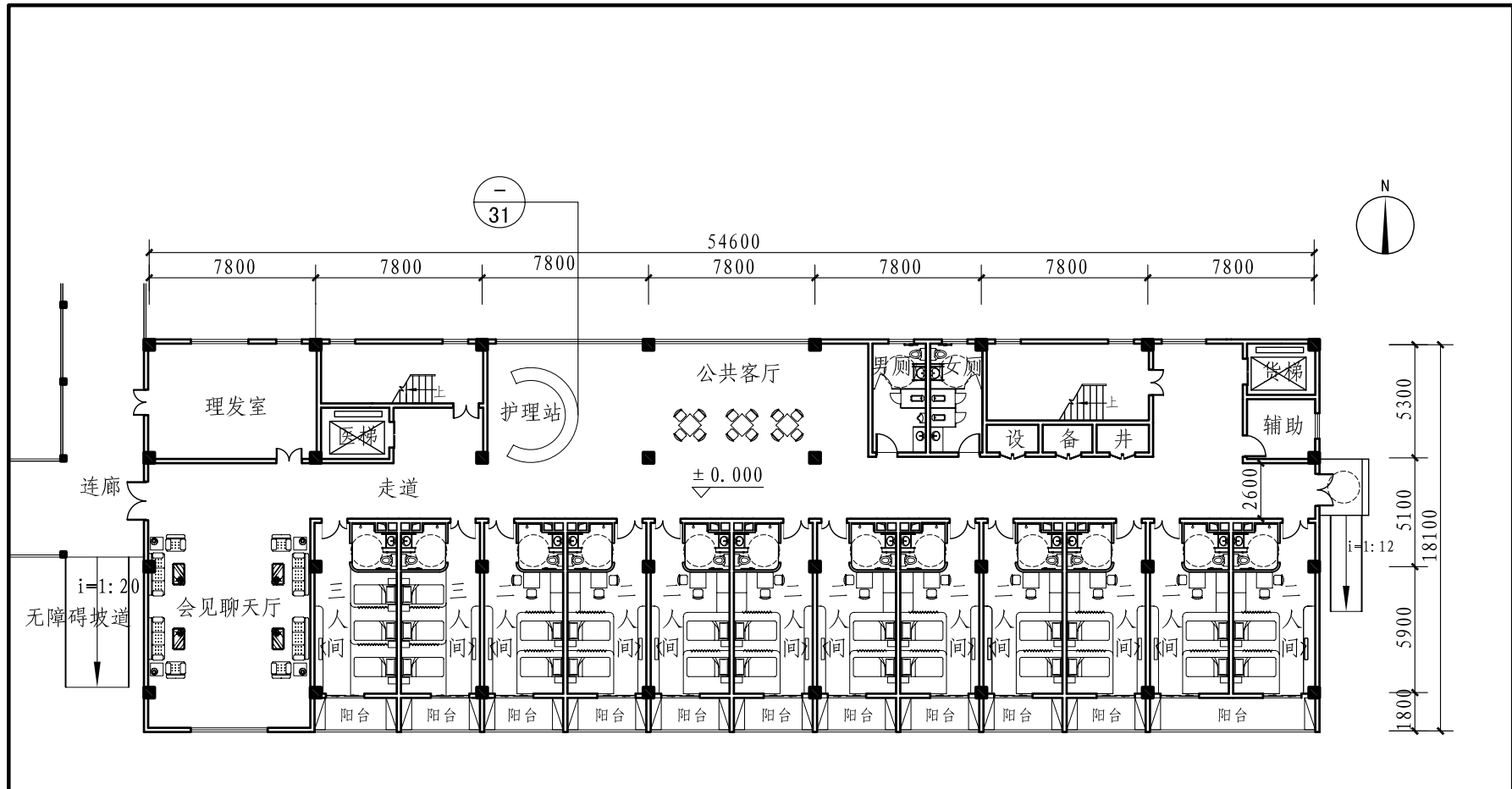
一层平面图
