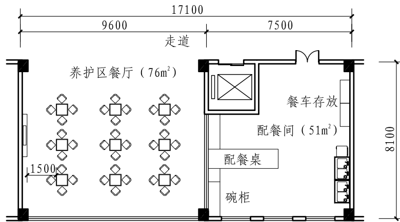
① 100床养护区餐厅、配餐间(127m 2 )
