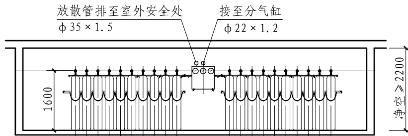
1-1 剖面
