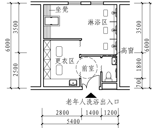
② 养护单元沐浴间
