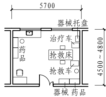
100床抢救室 (23.5m 2 )
