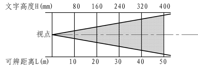
文字高度与可辨距离关系图
