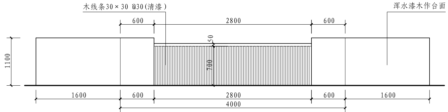
服务台展开立面图
