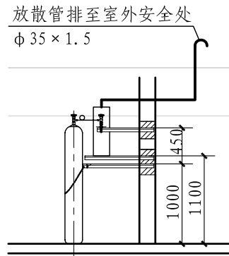
2-2 剖面
