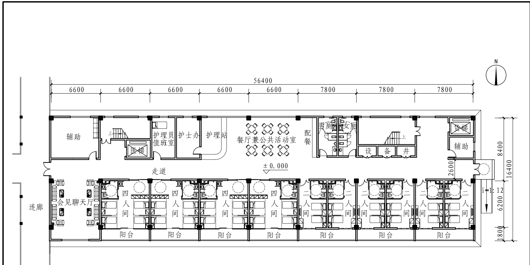
一层平面图
