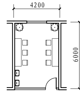
100床书画室 (23m 2 )
