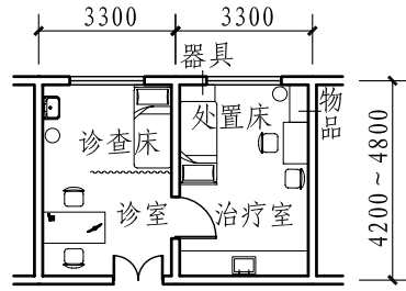
套间诊疗室(25m 2 )
