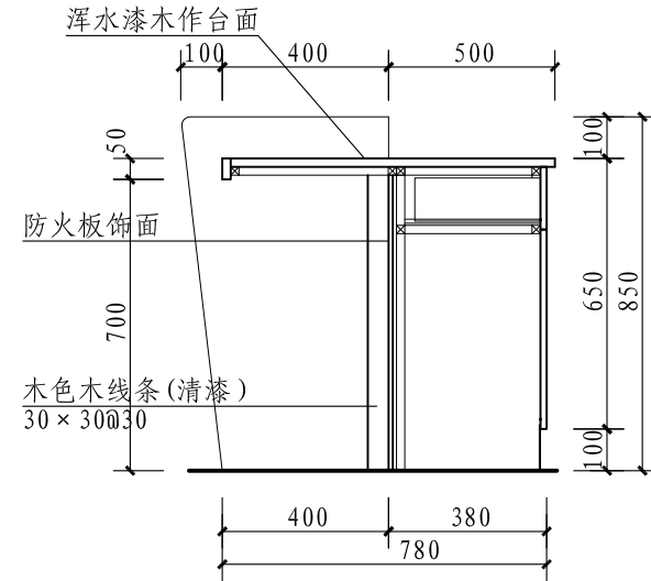
1-1 剖面图
