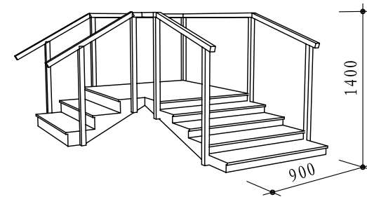
步态训练阶梯
