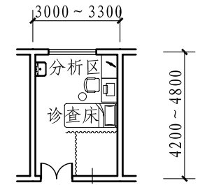
患者准备区 心电图室(11m 2 )
