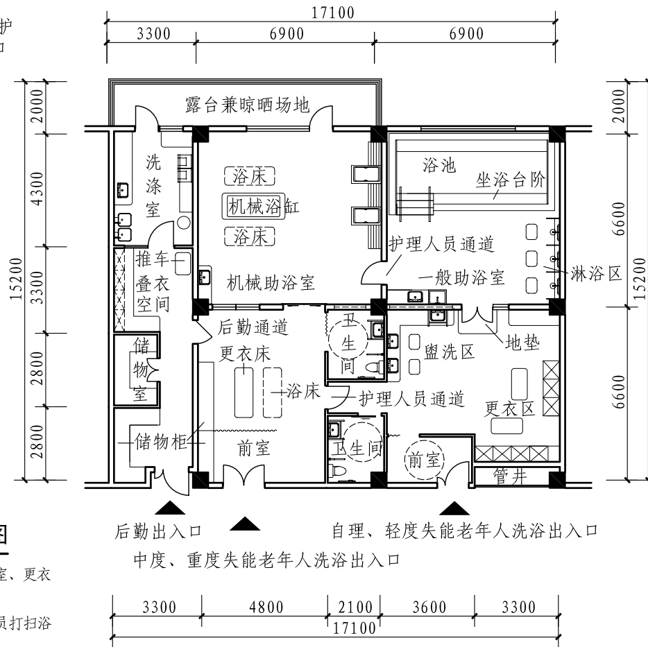
③ 集中沐浴间 (含一般助浴室和机械助浴室)
