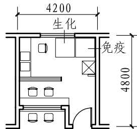
200、300床化验室(18m 2 )
