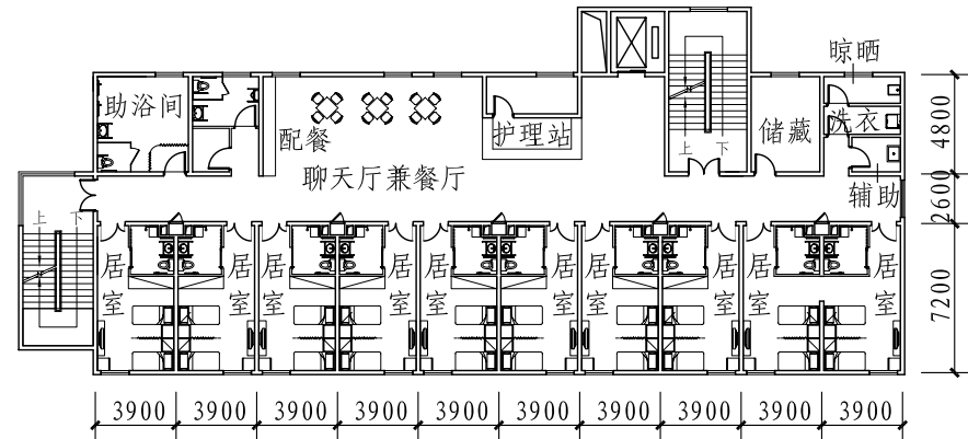
20床养护单元示意图
