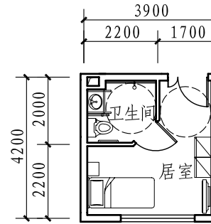
单人居室(二) (10.9m 2 )
