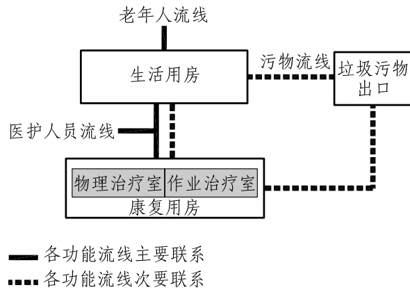
养护单元与康服用房关系框图
