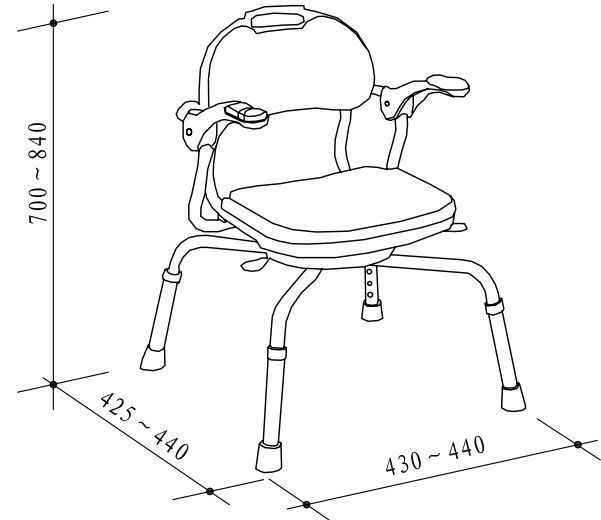
扶手式旋转洗澡椅
