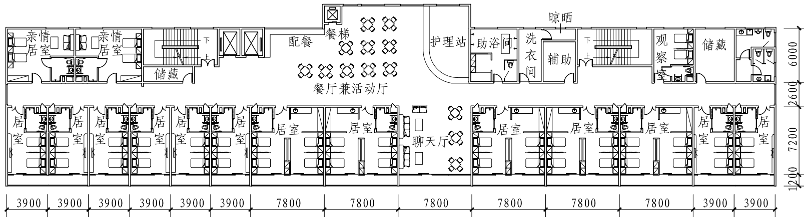
20床养护单元示意图
