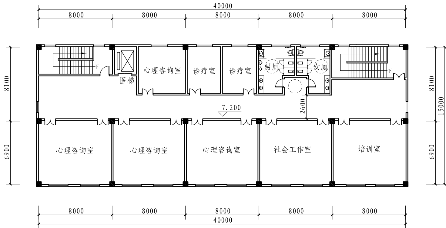
三层平面图
