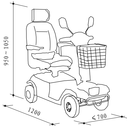
电动代步车立体关系
