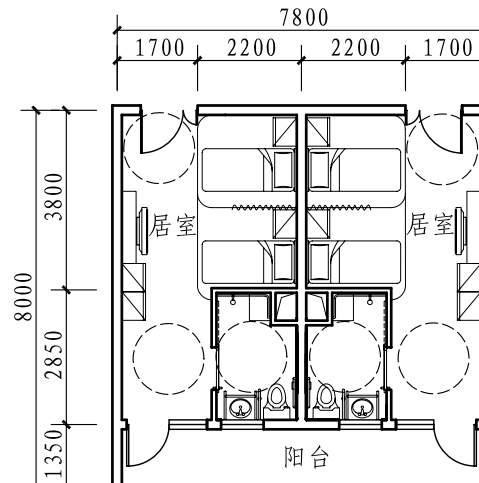
双人居室(三) (18.8m 2 )
