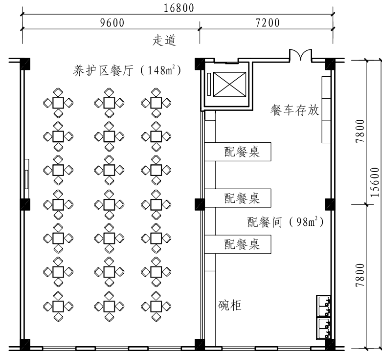
② 200床养护区餐厅、配餐间(246m 2 )
