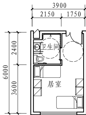
双人居室(一) (16.5m 2 )
