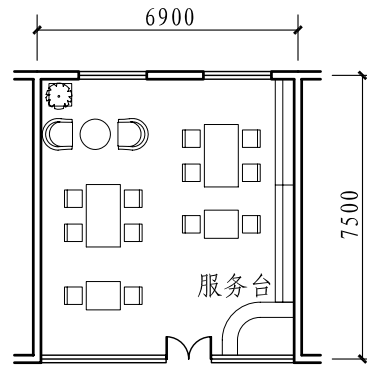
500床阅览室 (49m 2 )
