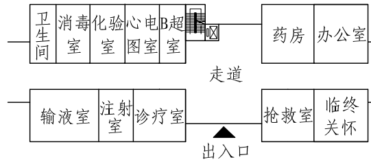
卫生保健用房平面布置示意图
