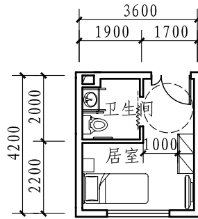
单人居室(一) (10.0m 2 )
