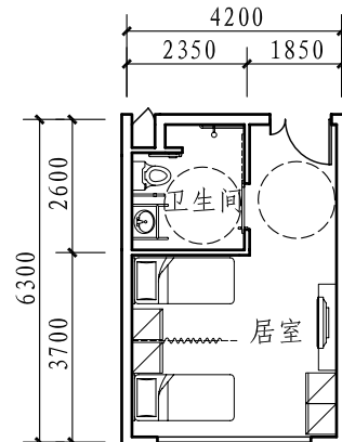
双人居室(二) (18.5m 2 )
