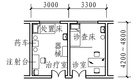
独立诊疗室(23.5m 2 )
