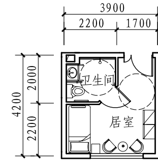
单人居室(三) (10.9m 2 )
